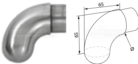
départ de main-courante crosse bout arrondi
