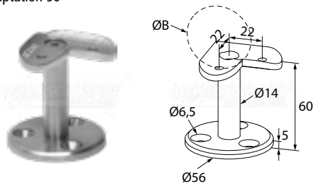
support de main-courante avec plaque d'adaptation 90°
