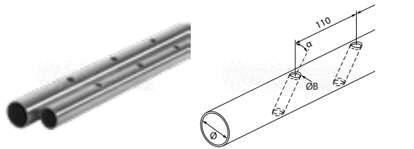
tube rond avec perforations traversantes
