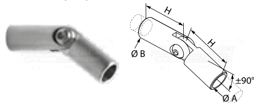
raccord articulé pour profils ronds
