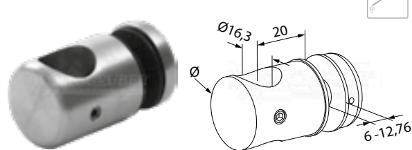
support de lisse pour verre
