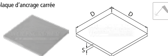
plaque d'ancrage carrée
