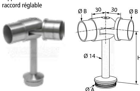
support de main-courante avec raccord réglable
