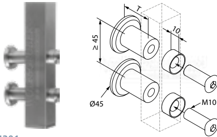
fixation murale (la paire) (info 1)
