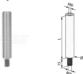
pivot avec filetage interne et externe
