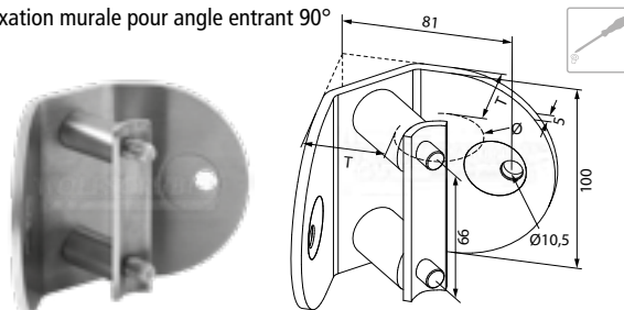
fixation murale pour angle entrant 90°
