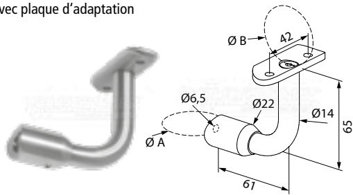
support de main-courante latéral avec plaque d'adaptation
