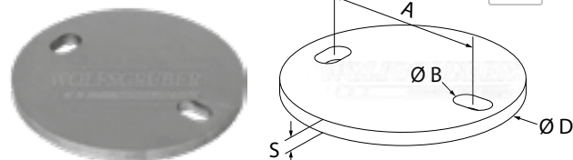
plaque d'ancrage avec 2 trous
