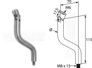
pivot articulé avec filetage interne et externe
