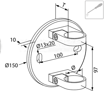
fixation murale à serrage
