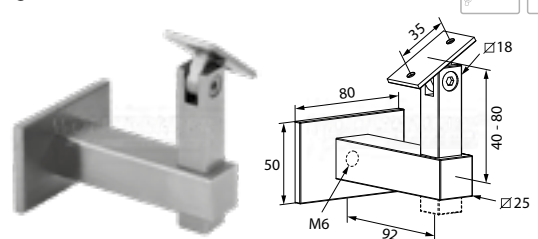
support de main-courante articulé avec platine et réglable en hauteur
