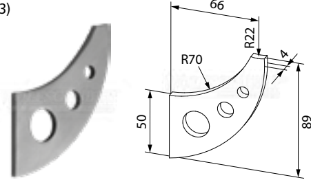
support de main-courante coupé au laser (info 3)
