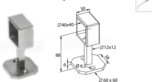
support de main-courante avec bague
