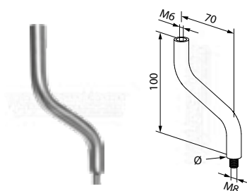
pivot avec filetage interne et externe
