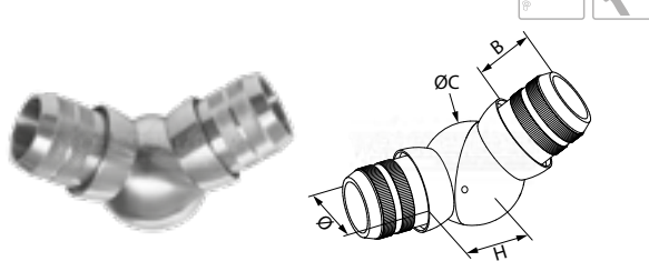
raccord d'angle orientable 90° - 180°
