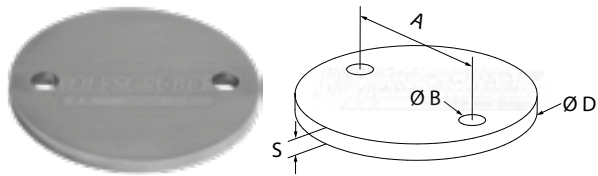
plaque d'ancrage avec 2 trous
