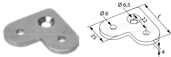
plaque d'adaptation main-courante 90° pour tubes carrés
