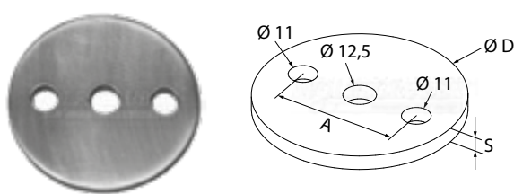
plaque d'ancrage avec 3 trous
