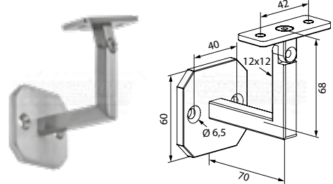
support de main-courante articulé avec plaque d'adaptation
