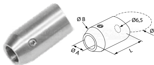
support de lisse pour pose dans l'axe
