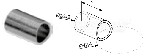
distanciateur
