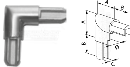
raccord d'angle pour cadre de remplissage rond
