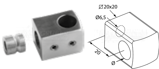
support de lisse avec trou passant
