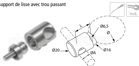
support de lisse avec trou passant
