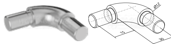
connecteur tube 90°
