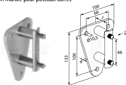
fixation murale pour poteaux carrés
