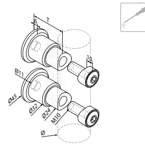
fixation murale (paire) réglable (info 1, 3)
