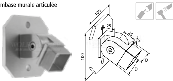
embase murale articulée
