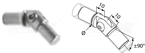
raccord articulé pour tubes
