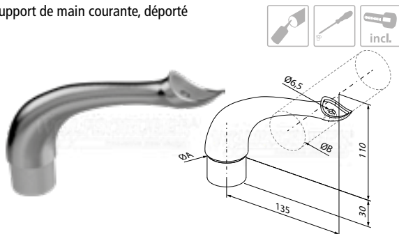
support de main courante, déporté
