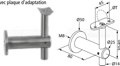
support de main-courante réglable en hauteur avec plaque d'adaptation
