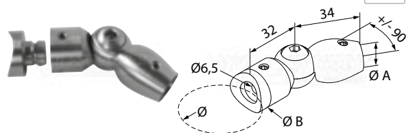
support de lisse articulé \pm 90^\circ
