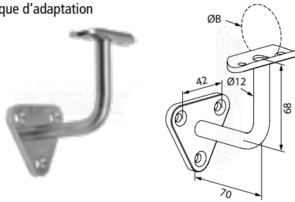
support de main-courante avec plaque d'adaptation
