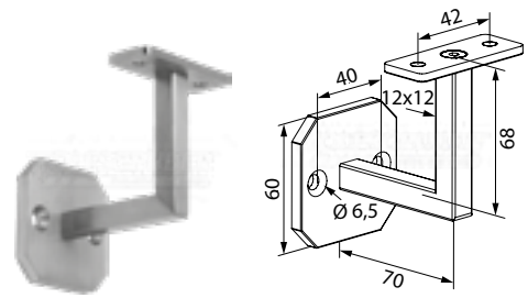
support de main-courante avec plaque d'adaptation
