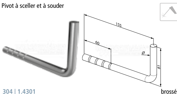
Pivot à sceller et à souder
