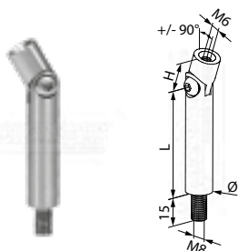
pivot articulé avec filetage interne et externe
