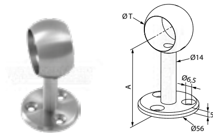
support de main-courante avec bague
