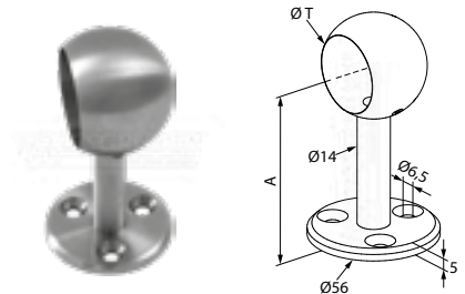
support de main-courante avec terminaison boule
