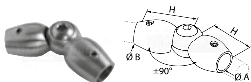
raccord articulé pour profils ronds
