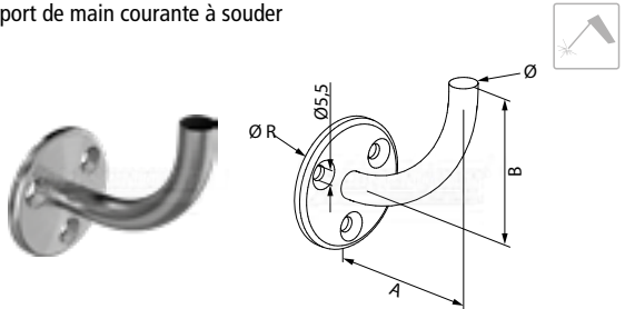
support de main courante à souder
