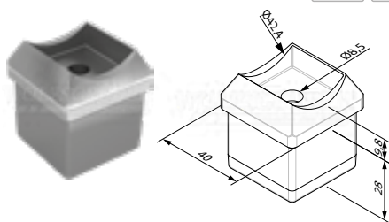
adaptateur (info 1)
