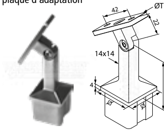
support de main-courante articulé avec plaque d'adaptation
