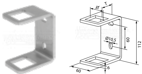
fixation murale découpe laser
