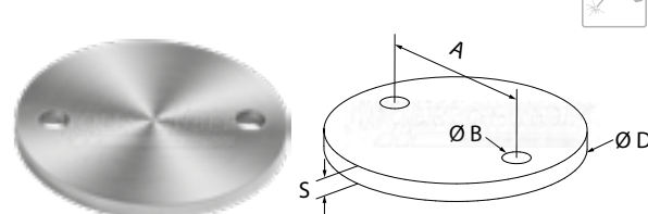
plaque d'ancrage avec 2 trous
