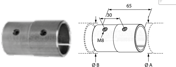
adaptateur avec vis de blocage
