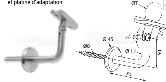
support de main courante avec articulation et platine d'adaptation
