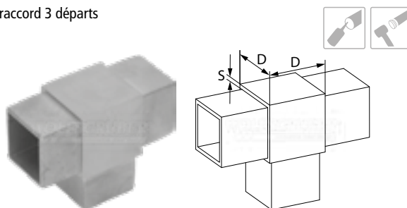
raccord 3 départs
