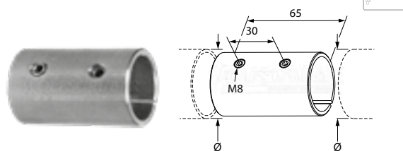
raccord avec vis de blocage
