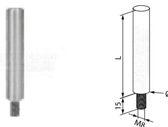
pivot avec filetage externe
