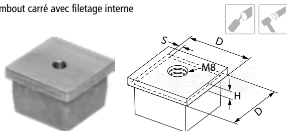
embout carré
