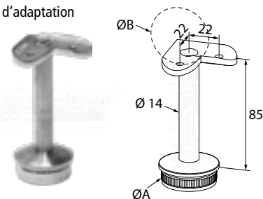
support de main-courante avec plaque d'adaptation
