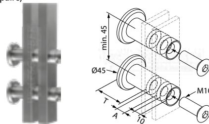
fixation murale pour poteau à double profilé plat (la paire)
