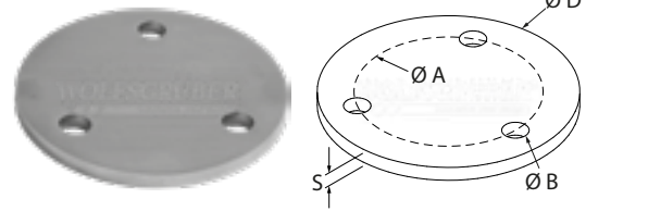
plaque d'ancrage avec 3 trous
