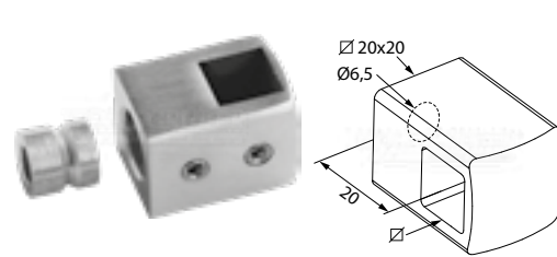
support de lisse avec trou passant
