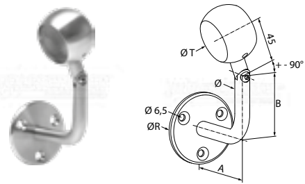
support de main-courante articulé avec bague
