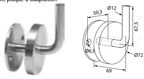
support de main-courante avec cache-embase sans plaque d'adaptation
