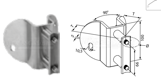
fixation murale pour angle sortant 90°
