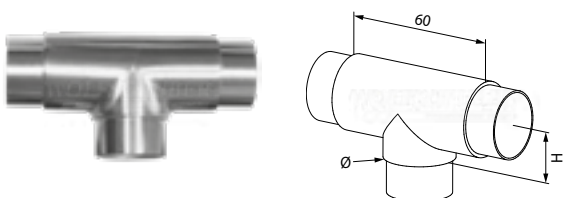
adaptateur tube sur tube (info 2)
