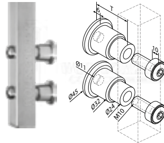
fixation murale (la paire) réglable (info 1 2)
