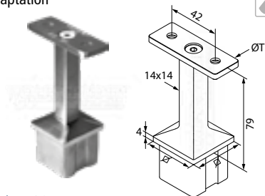
support de main-courante avec plaque d'adaptation
