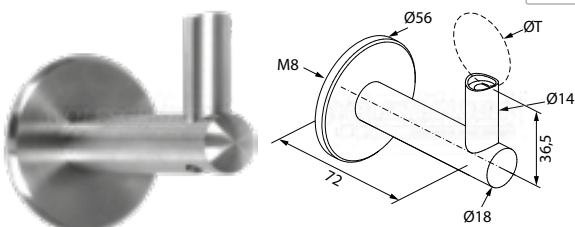
support de main-courante sans plaque d'adaptation
