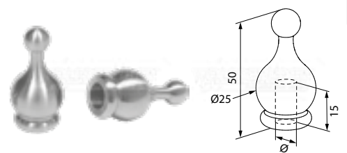
terminaison décorative
