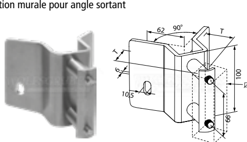
fixation murale pour angle sortant
