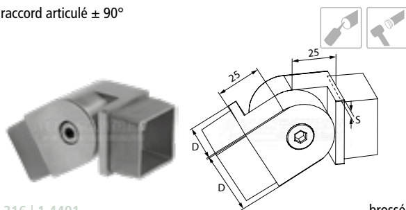
raccord articulé ± 90°
