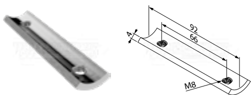
platine de fixation allant à l'intérieur du tube
