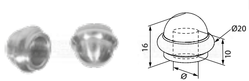
terminaison décorative
