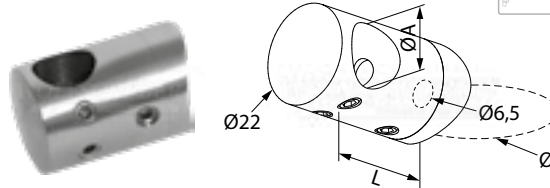
support de lisse avec trou passant (info 1)
