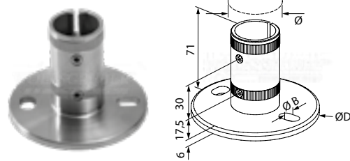
fixation au sol
