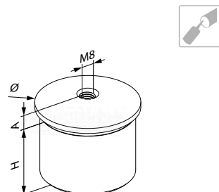
embout bombé à filetage interne
