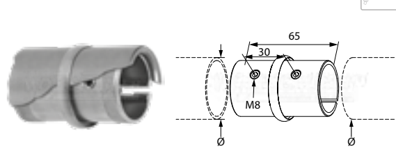
raccord de jonction avec bague et vis de blocage
