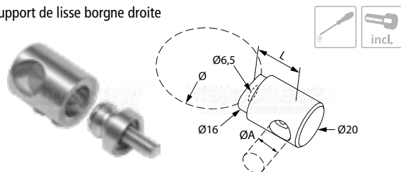
support de lisse borgne droite
